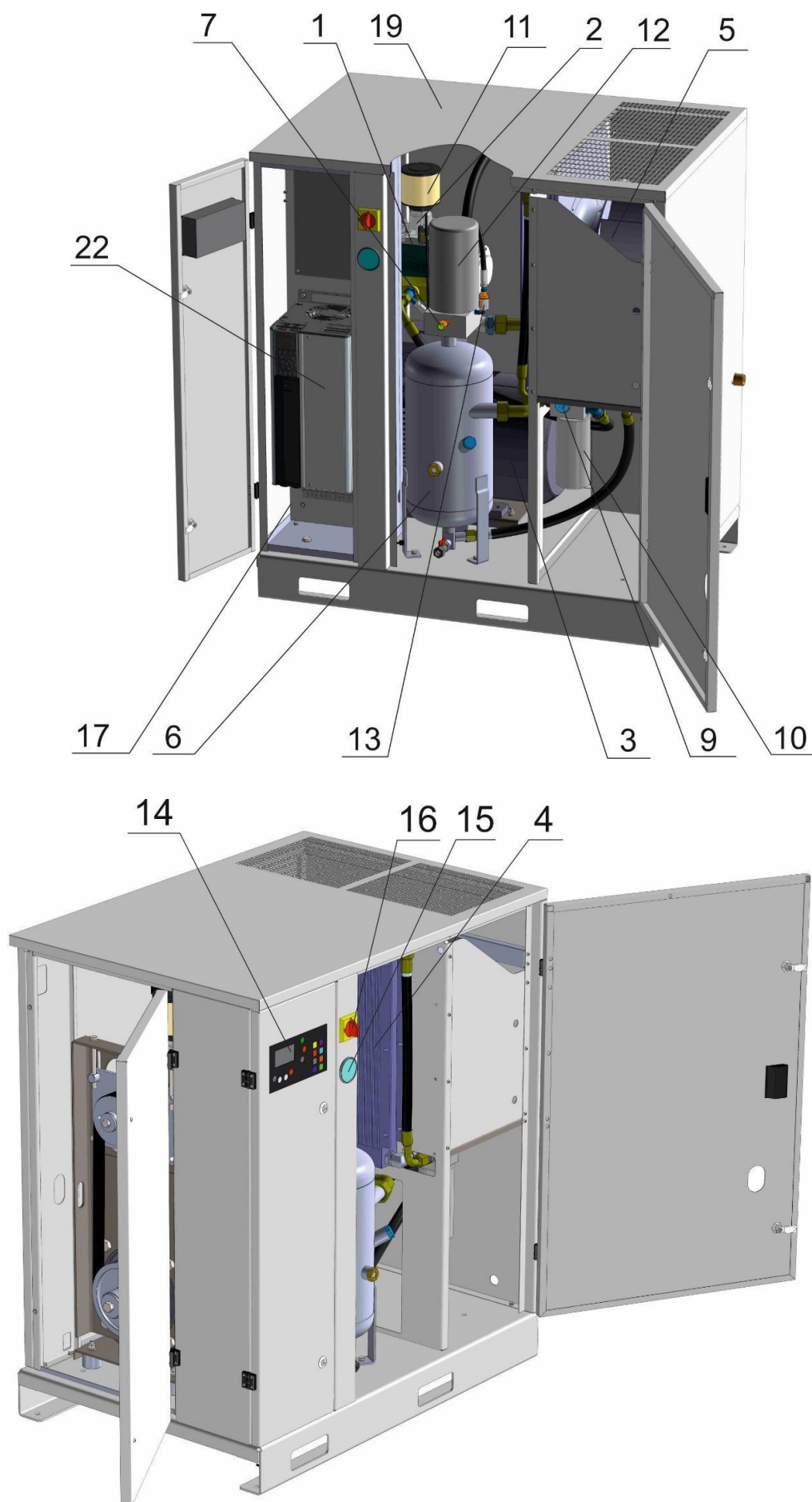
Рисунок 1 – Общий вид компрессорной установки BK25-...(BC), 30-...(BC)
